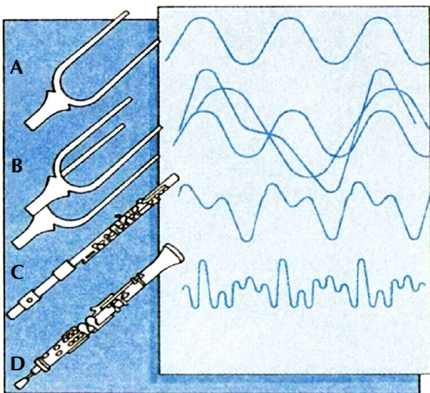
рис.1 Гармоники
