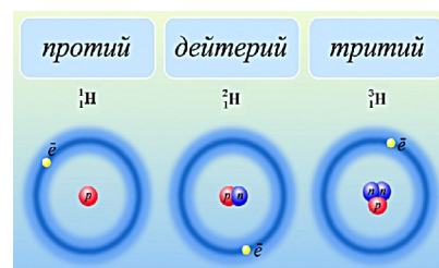
Изотопы водорода
