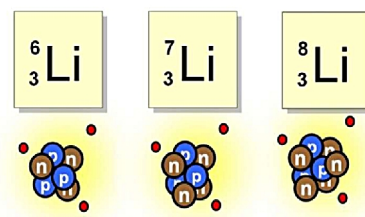
Изотопы лития
